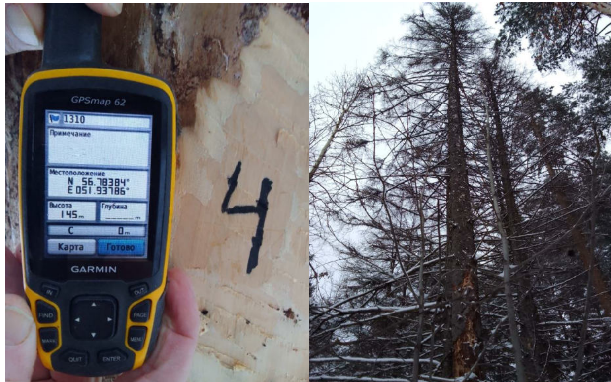
Аварийное дерево №4
