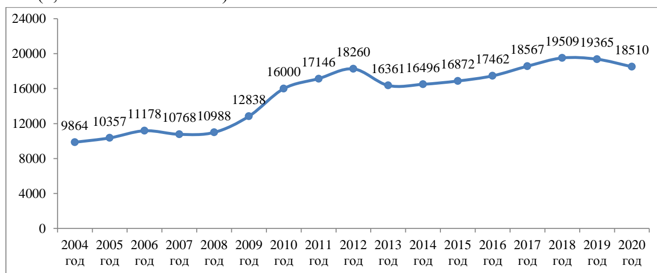
Рис. 1. Динамика численности лося в Удмуртской Республике по данным государственного мониторинга в период с 2004 по 2020 гг.
