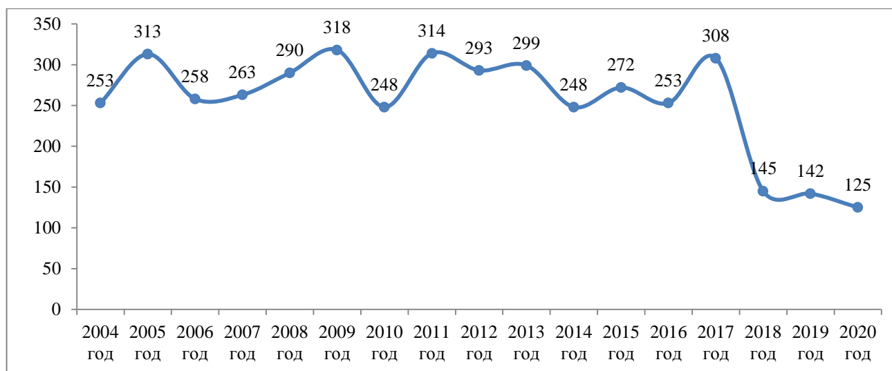
Рис. 3. Динамика численности рыси в Удмуртской Республике по данным государственного мониторинга в период с 2004 по 2020 гг.
